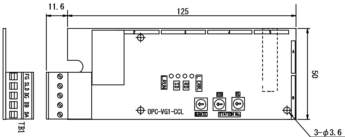
図 1.2-1 インタフェースカード外形
